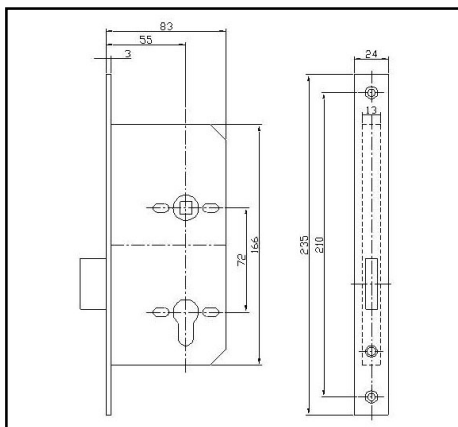
Backset 55 x c.c. 72 mm
