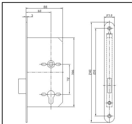
Backset 60 x c.c. 72 mm
