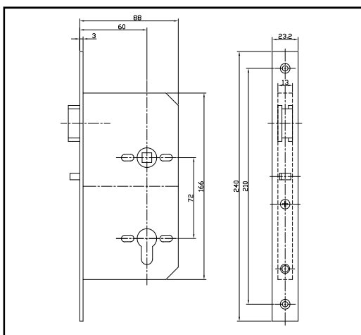
Backset 60 x c.c. 72 mm
