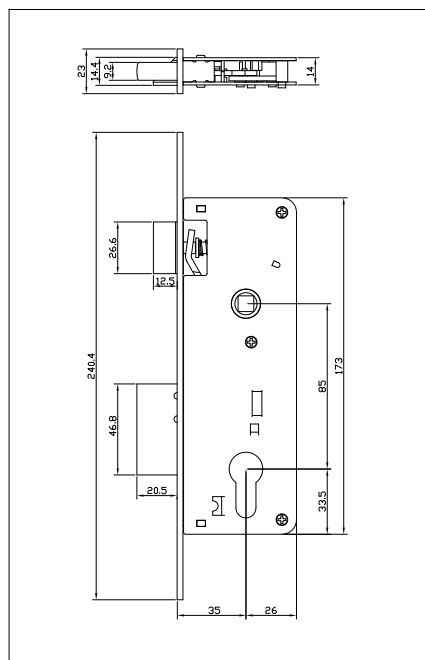
Backset 35 x c.c. 85 mm
