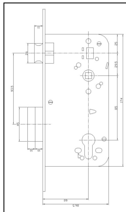
Backset 60 x c.c. 85 mm
