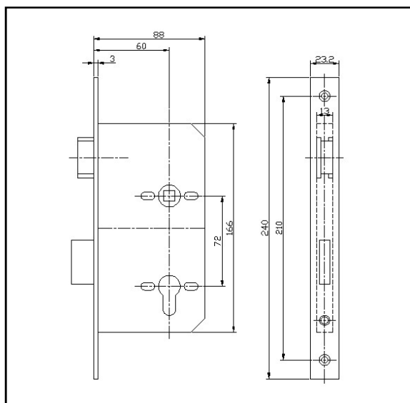
Backset 60 x c.c. 72 mm
