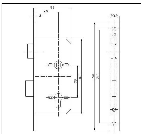
Backset 60 x c.c. 72 mm
