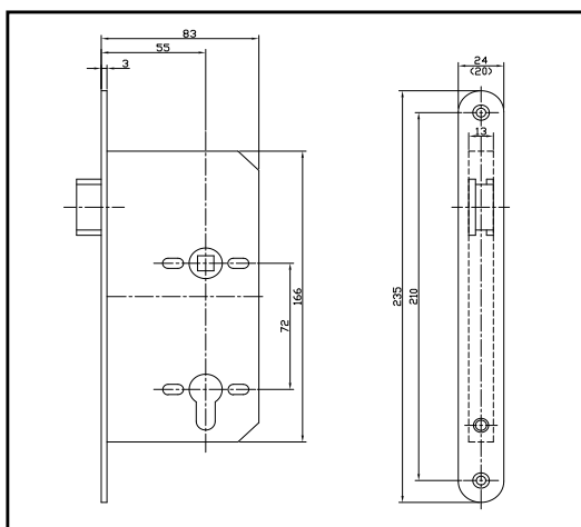
Backset 55 x c.c. 72 mm
