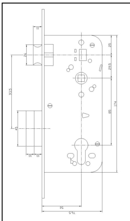
Backset 50 x c.c. 85 mm
